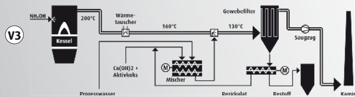
Abb. 1: Anlagenkonfiguration mit SCR (Referenzszenario) und SNCR-Verfahren (Alternativszenario)
